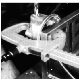
Carver T285-18 vpenjalna zobata letev v napravi za vrtnanje
