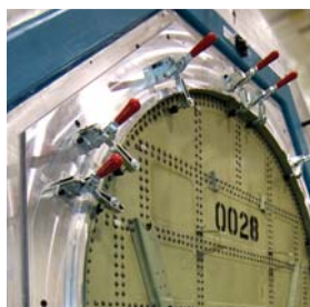
Model 207-U Navpično vpenjalo v montažni napravi za letalske celice
