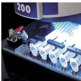
Model 305-U Kompaktno vodoravno vpenjalo v napravi za izdelovanje za medicinske izdelke
